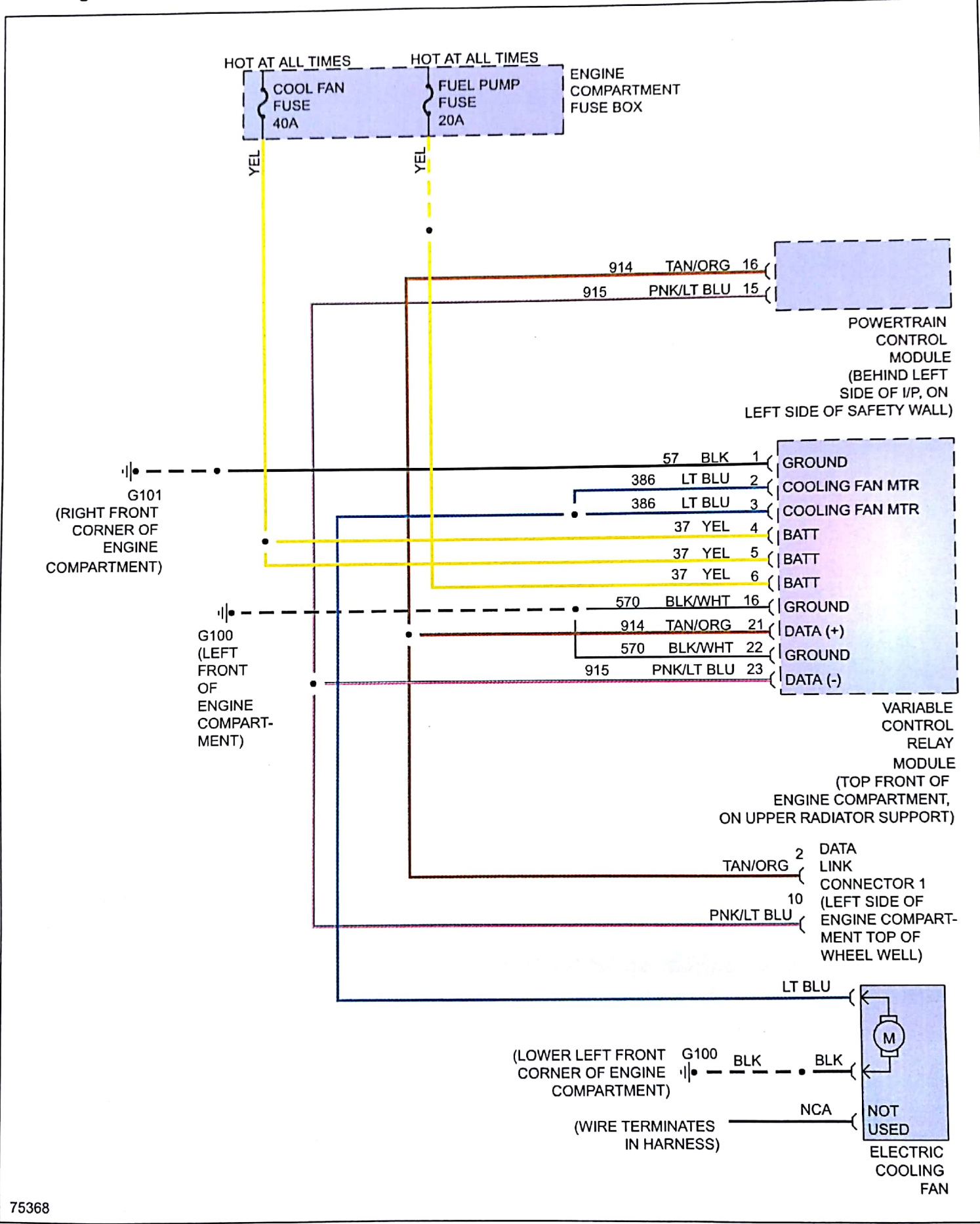
Fig 1: Cooling Fan Circuit
